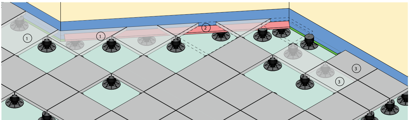
Fig. 8: Disposition des plots sous les dalles coupées; (1) dalles coupées, variante avec un format de dalle plus grand, (2) profilé en métal, (3) raccordement réparti sur 2 ou 3 rangées de dalles de même largeur
