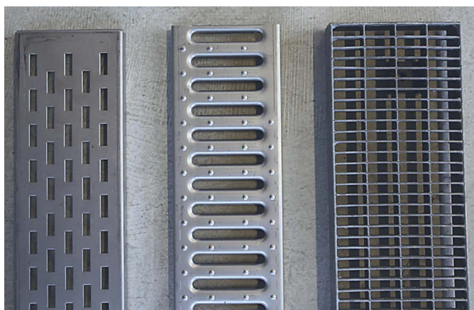
Fig. 15: Grille perforée (à gauche), à passerelles (milieu), caillebotis (à droite)
